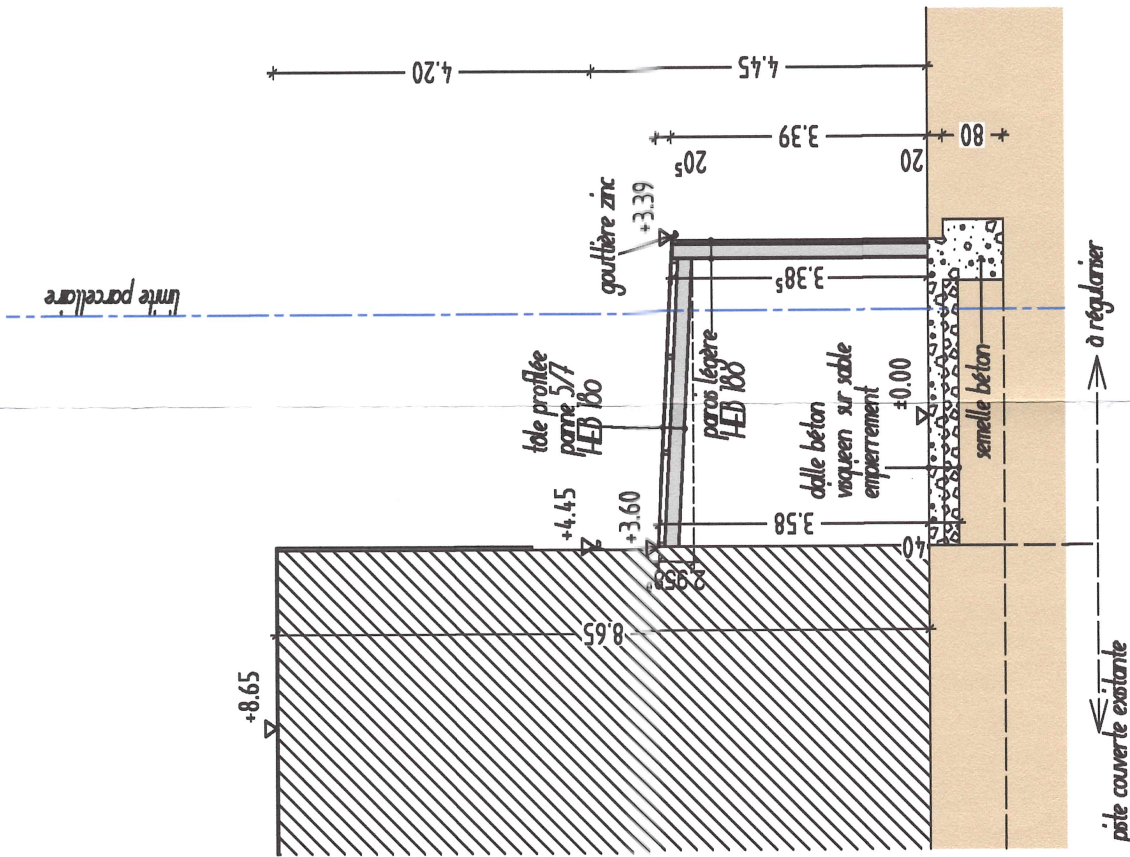
COUPE C - C'
