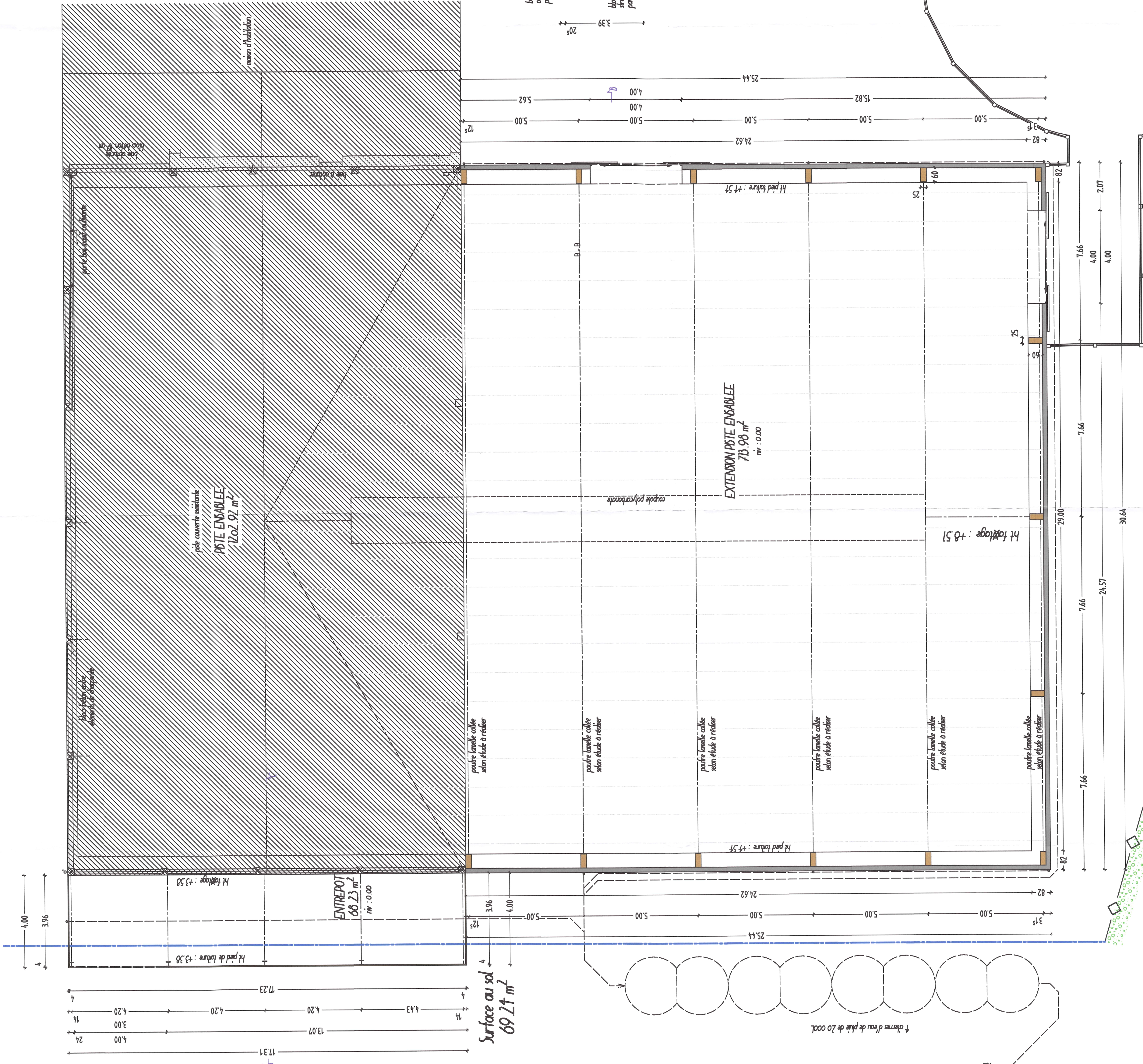
VUE EN PLAN
