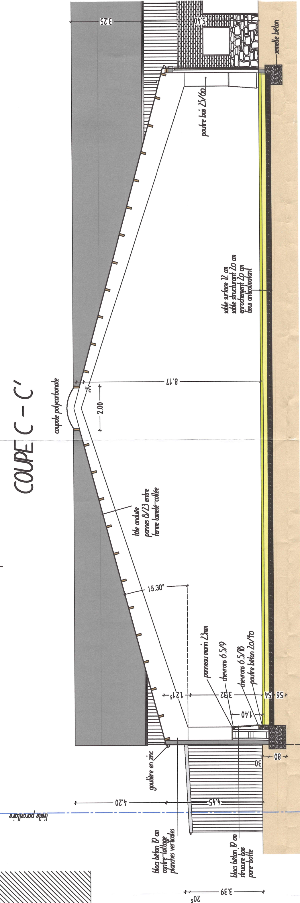
COUPE B - B'
